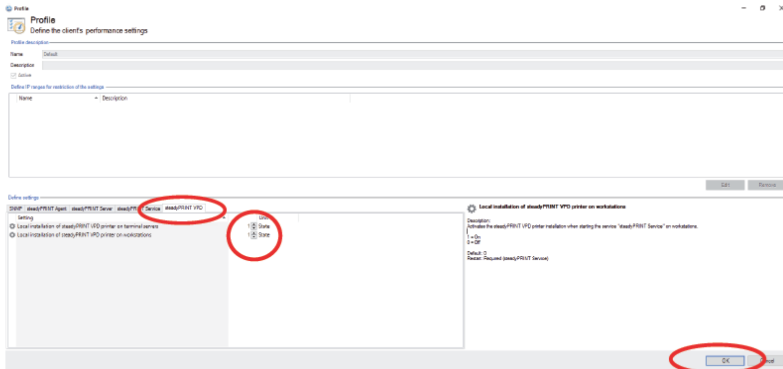
Abbildung 238: Im Tab "steadyPRINT VPD" beide Werte auf "1" setzen und anschließend mit OK bestätigen
