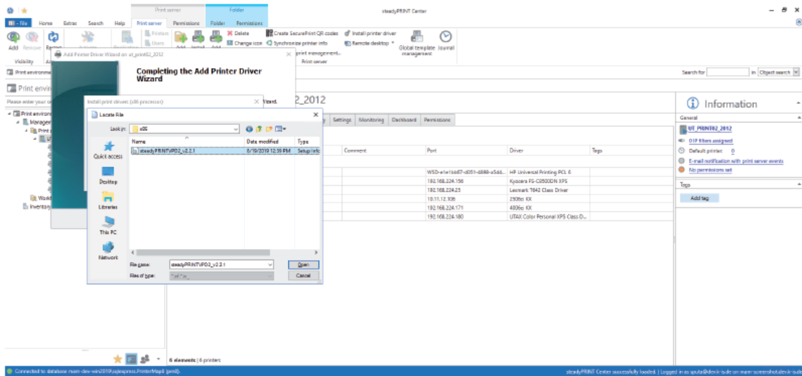
Abbildung 232: Wählen Sie den Treiber aus dem Ordner „Virtual Printer Driver“ im steadyPRINT-Installationsverzeichnis aus.
