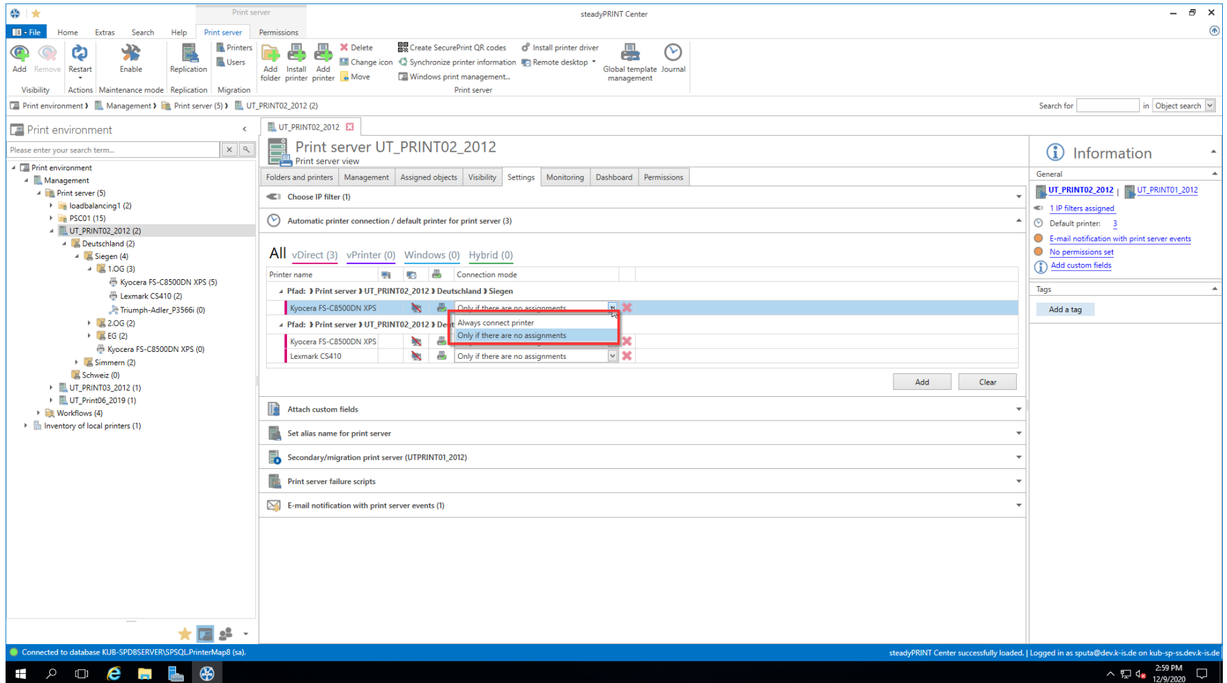
Abbildung 31: steadyPRINT Center: Individualisierung automatischer Druckerverbindungen
