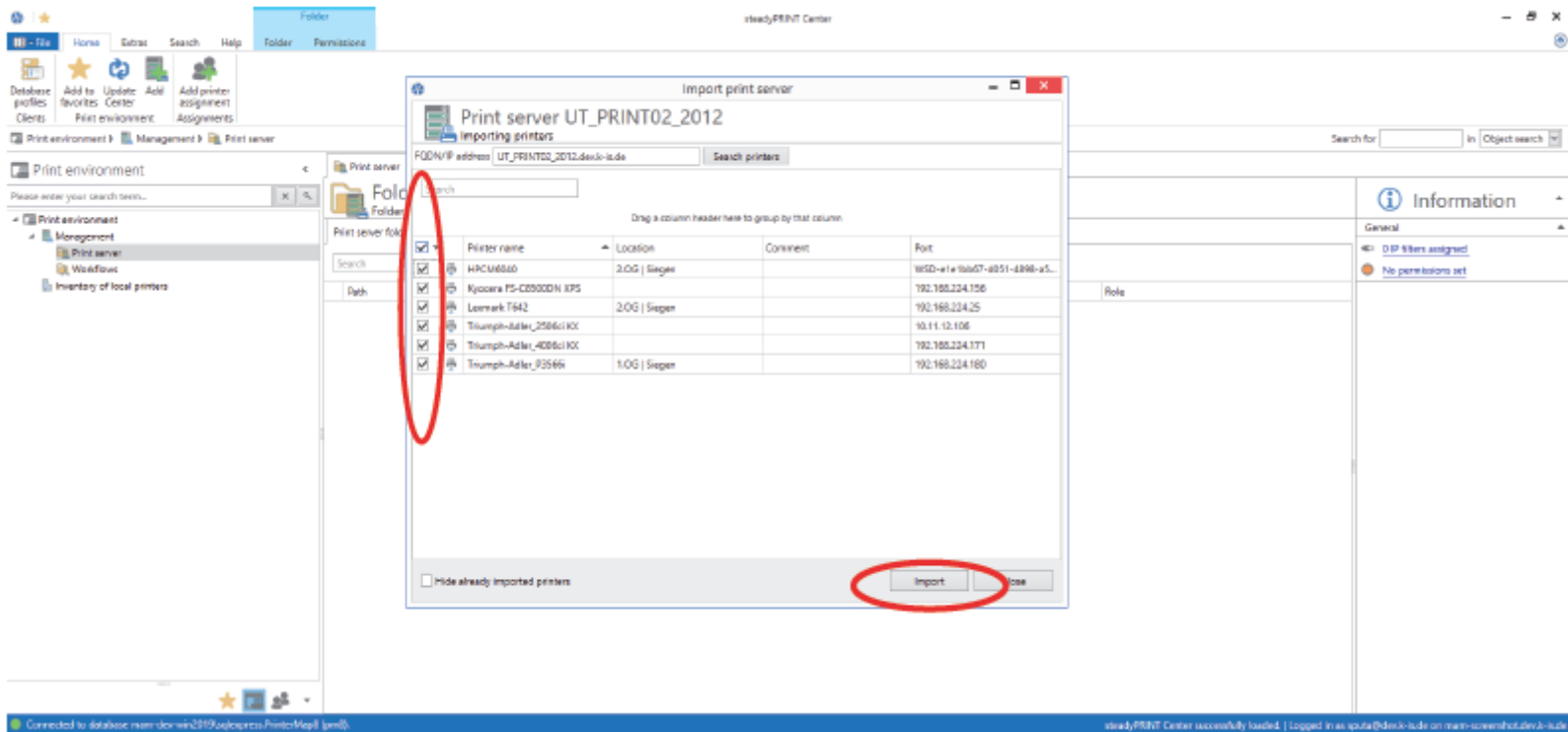
Abbildung 219: Drucker auswählen &amp; importieren
