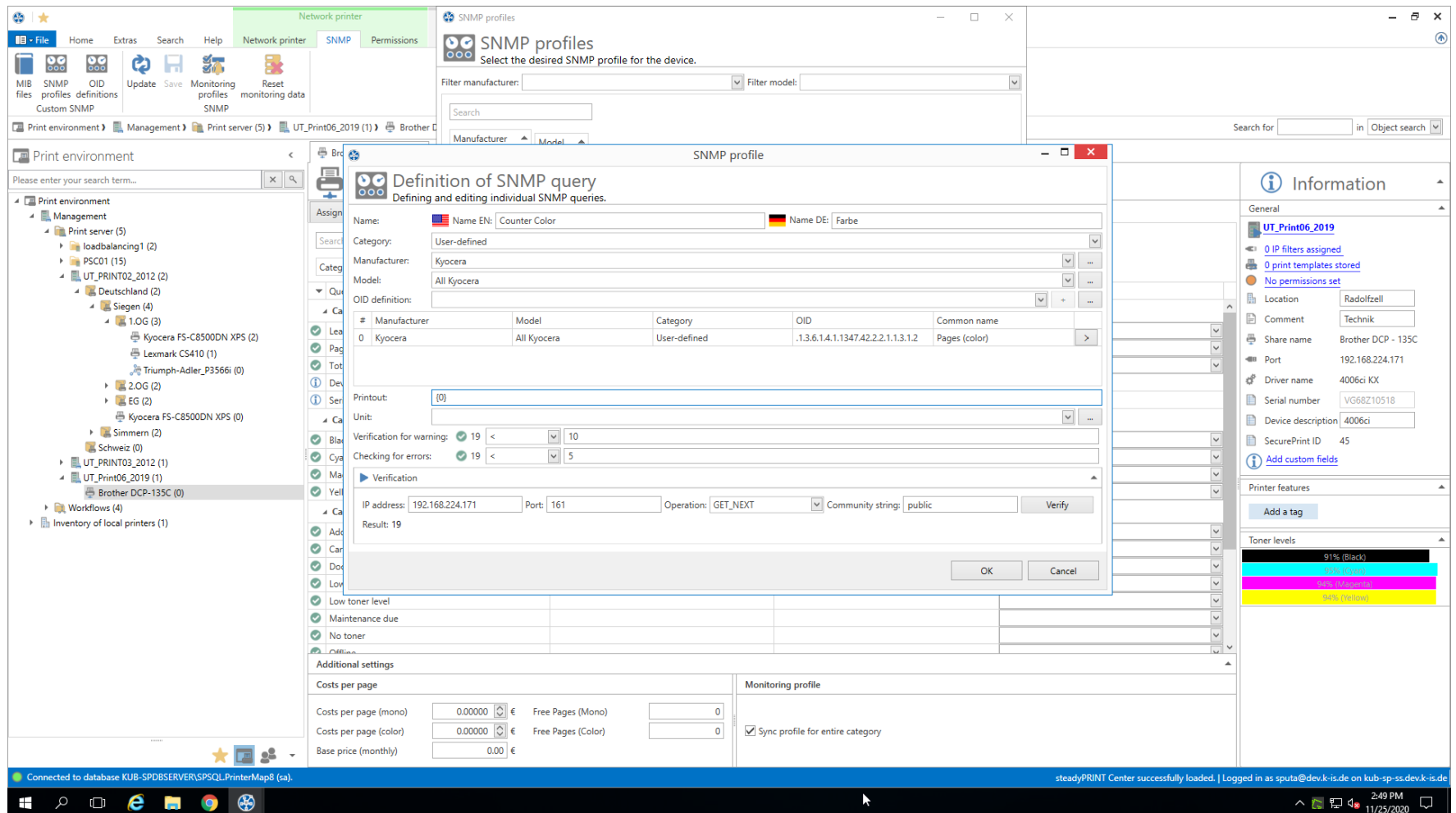
Abbildung 142: steadyPRINT Center - SNMP-Abfrage fehlgeschlagen (Ausdruck fehlerhaft)
