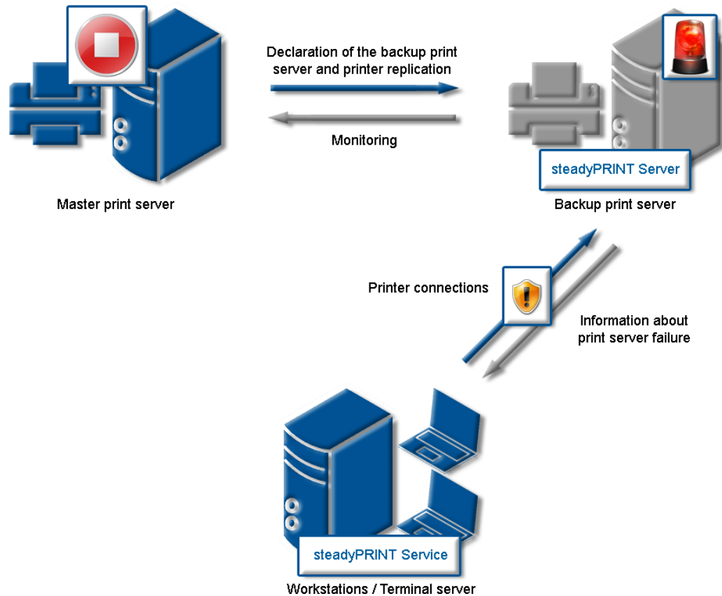
Abbildung 155: Nach dem Ausfall des Master-Druckerservers
